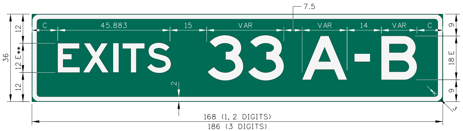
E1-5P EXIT NUMBER (PLAQUE)
