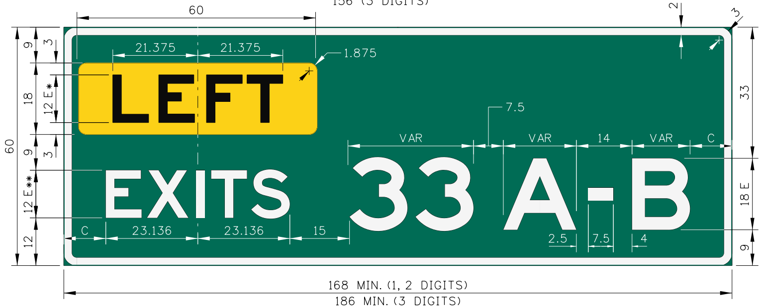
E1-5bP LEFT EXIT NUMBER (PLAQUE)
