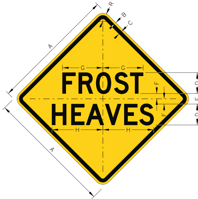
W8-801 FROST HEAVES
