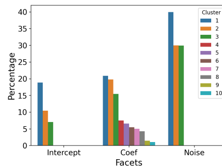
(d) \pi for facets
