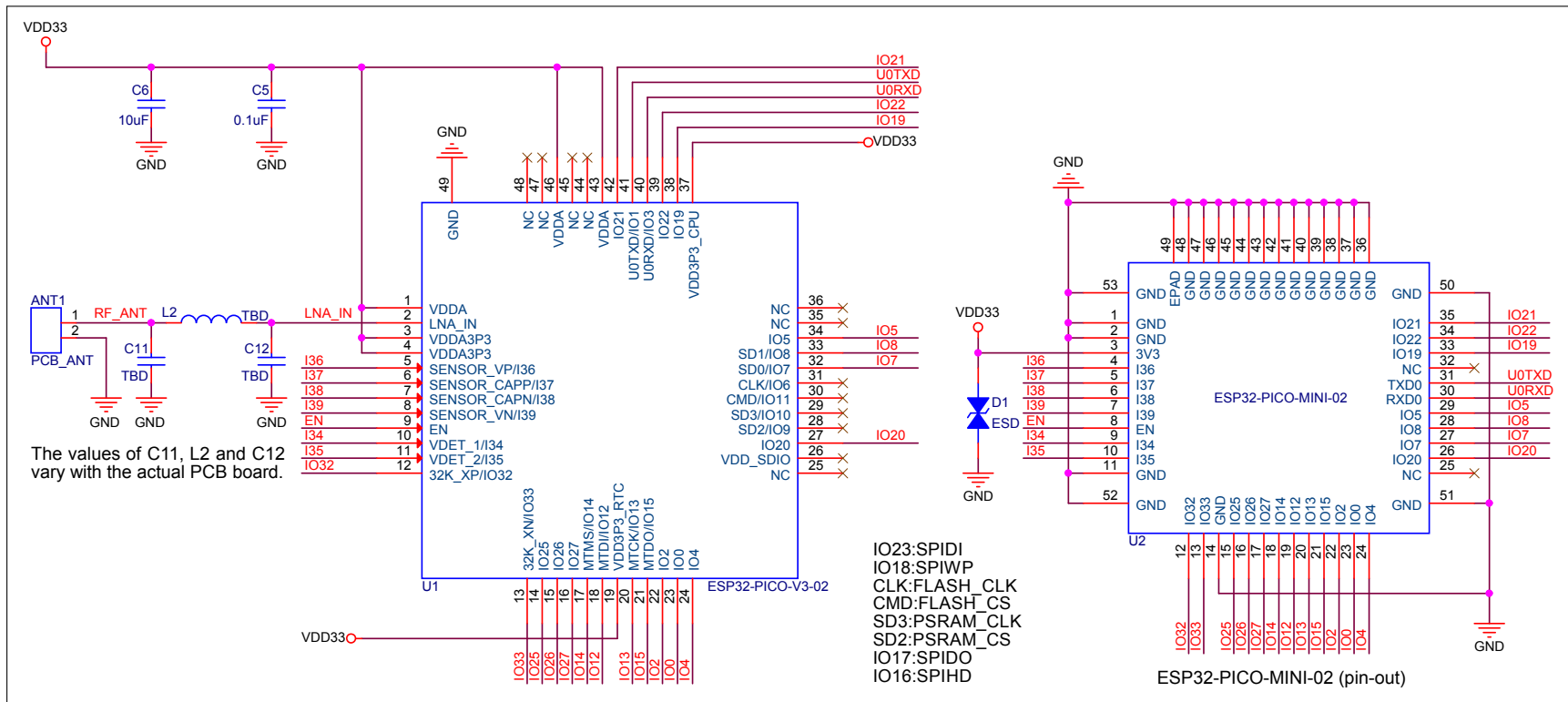
图 8: ESP32-PICO-MINI-02 原理图
