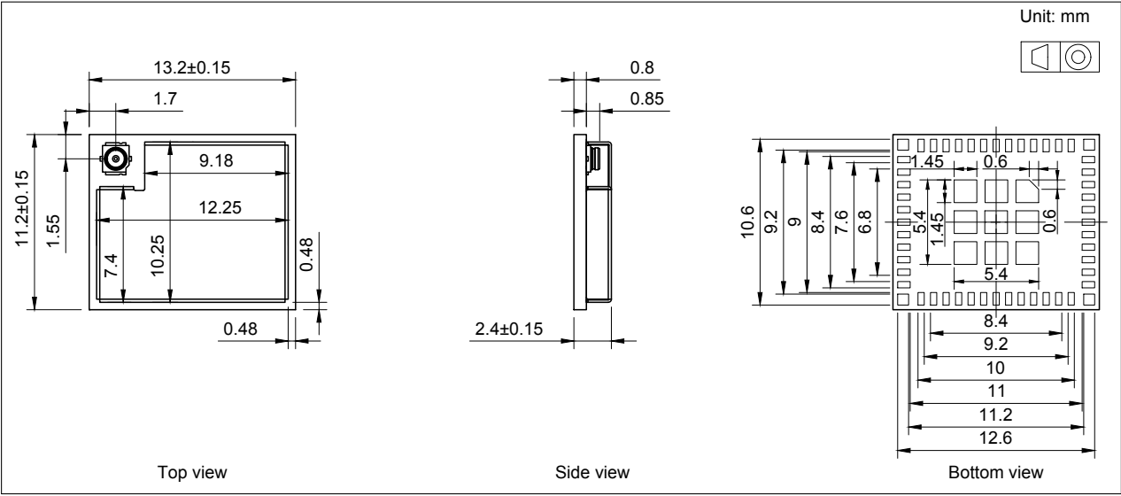
图 12: ESP32-PICO-MINI-02U 模组尺寸
