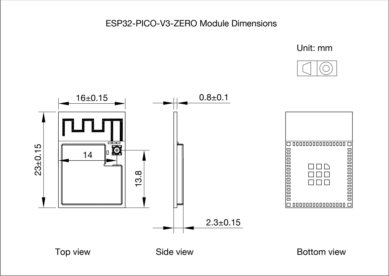
图 7: 模组尺寸
