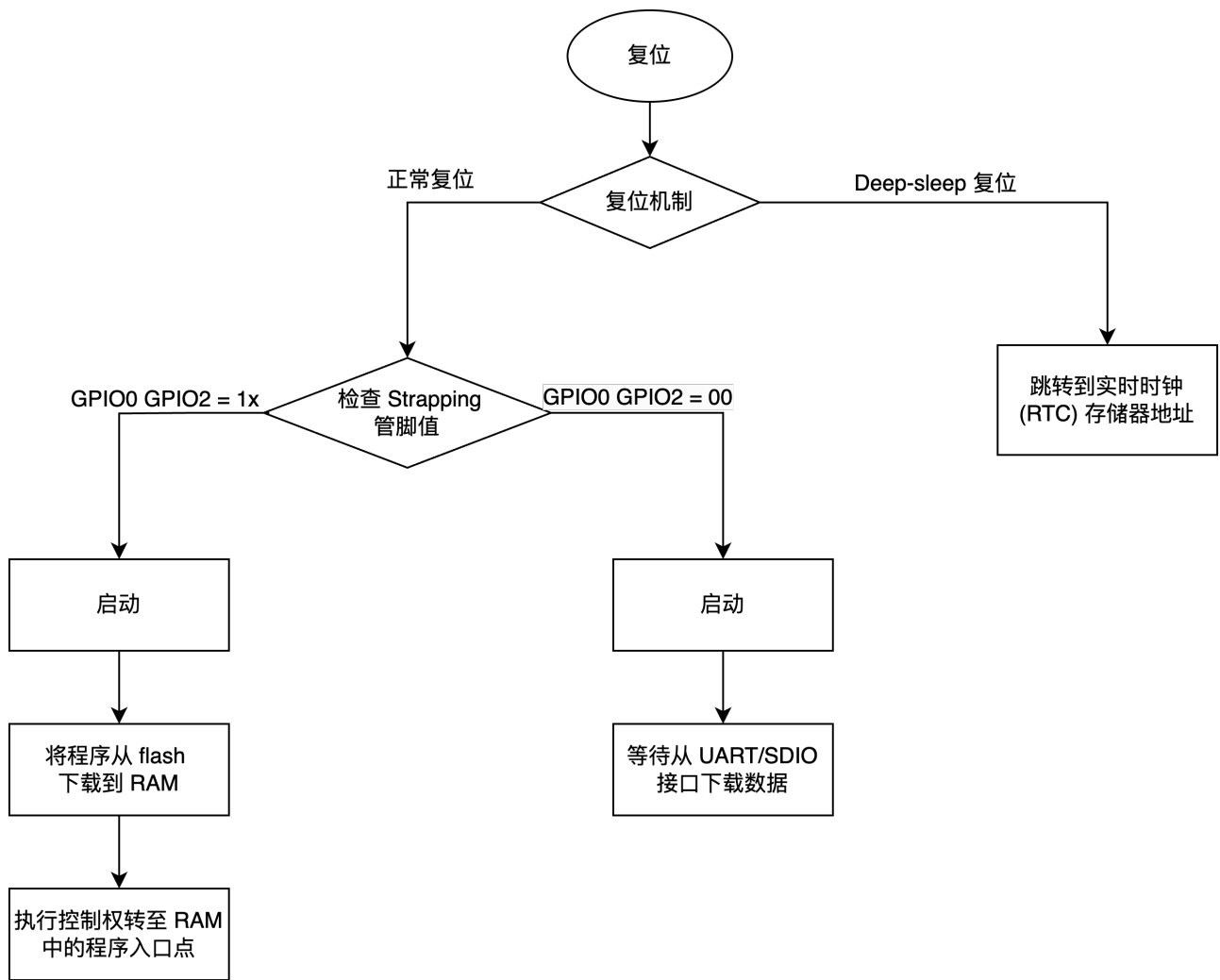
图 4: 芯片启动流程
