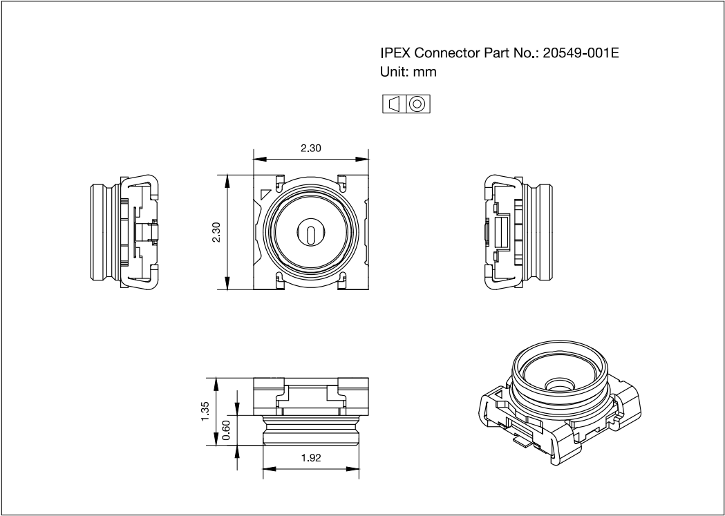
图 11: RF 测试连接器尺寸
