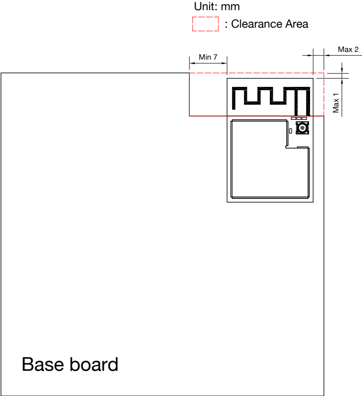
图 10: 天线区域净空示意图
