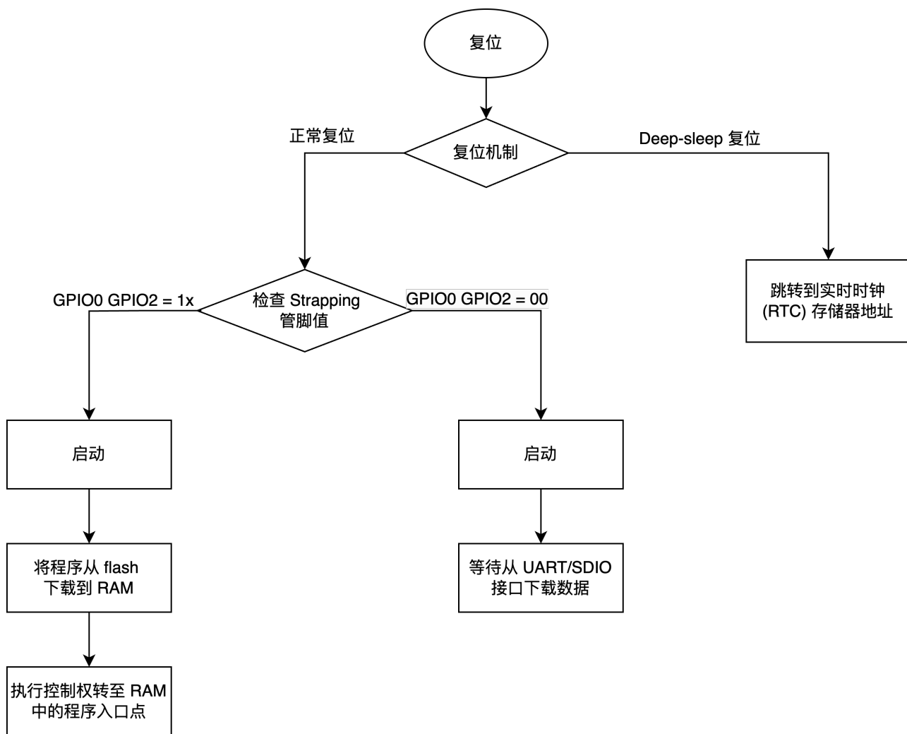
图 3: 芯片启动流程
