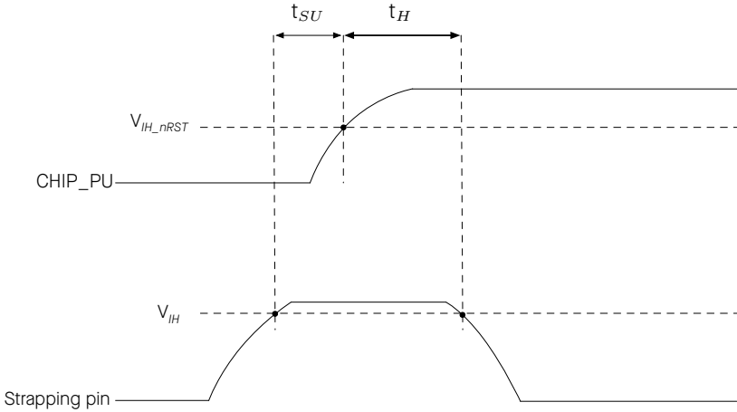
图 2: Strapping 管脚的时序参数图
