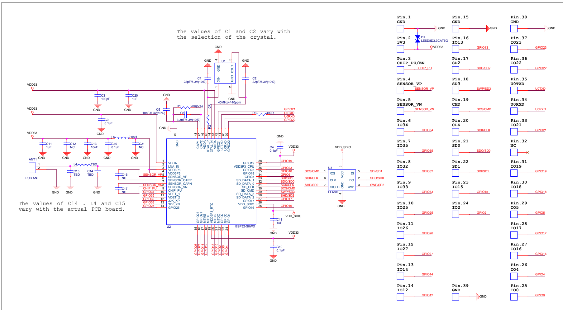
图 5: ESP32-SOLO-1 原理图
