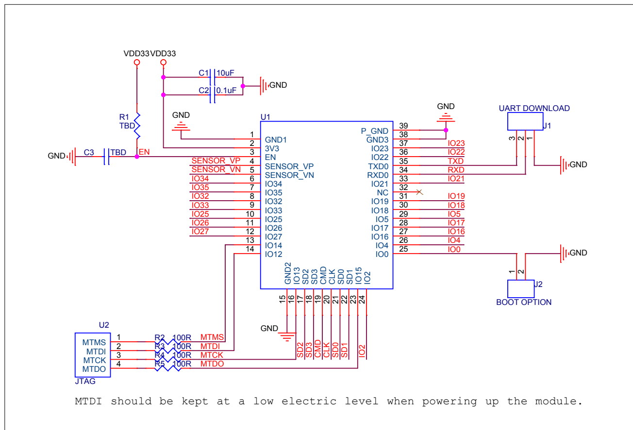
图 6: 外围设计原理图
