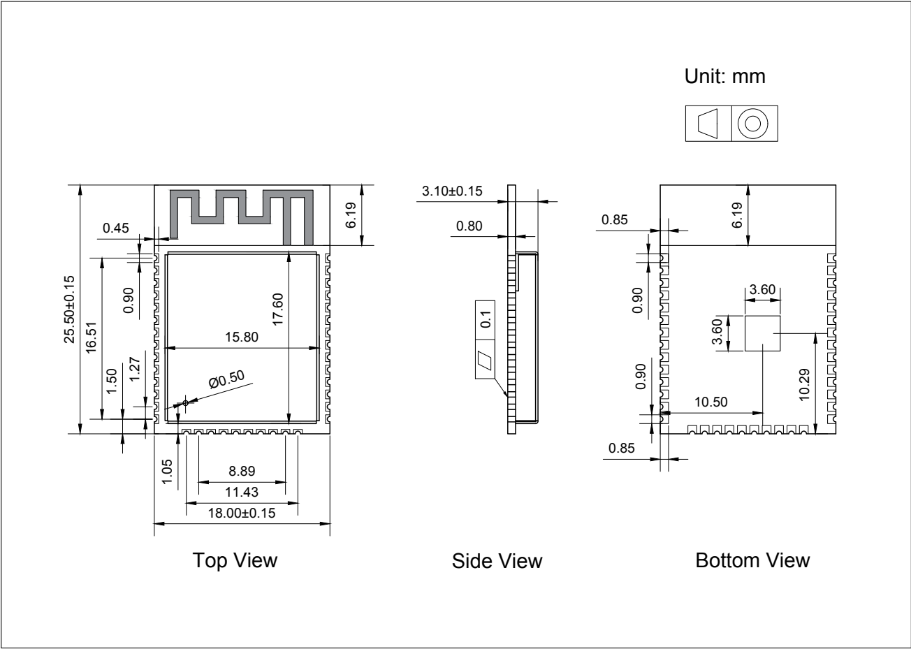
图 7: 模组尺寸
