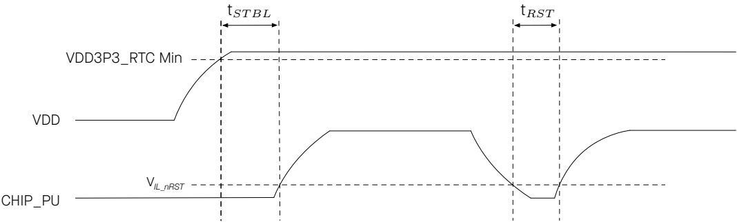
图 4: 上电和复位时序参数图
