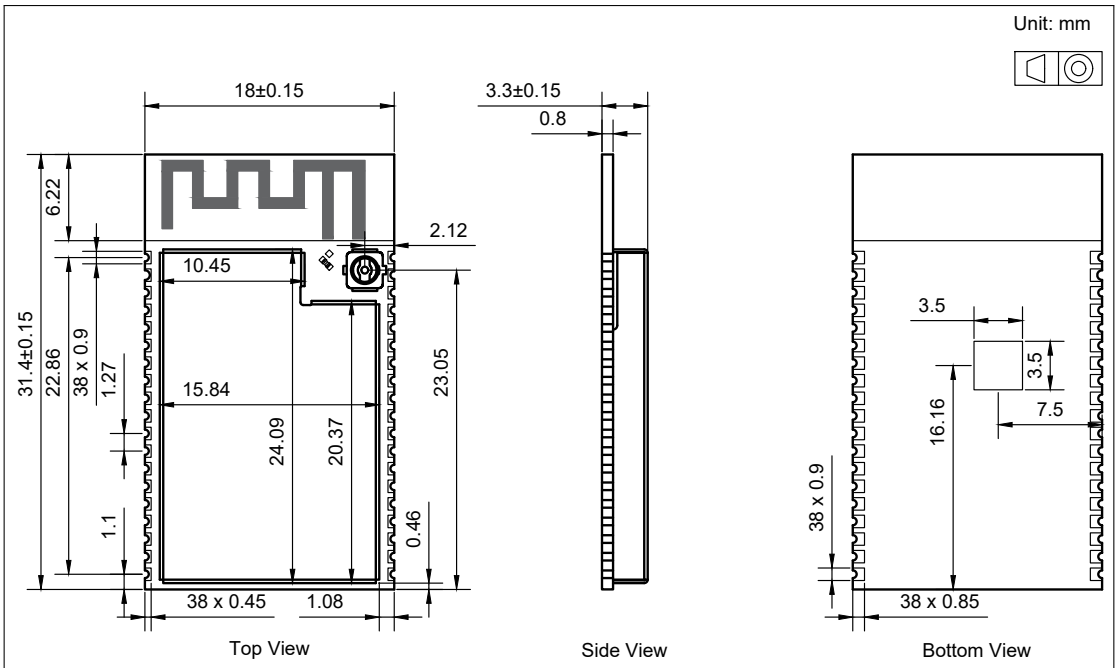
图 9: ESP32-WROVER-IB 模组尺寸
