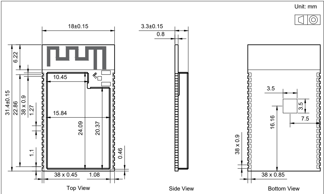
图 8: ESP32-WROVER-B 模组尺寸
