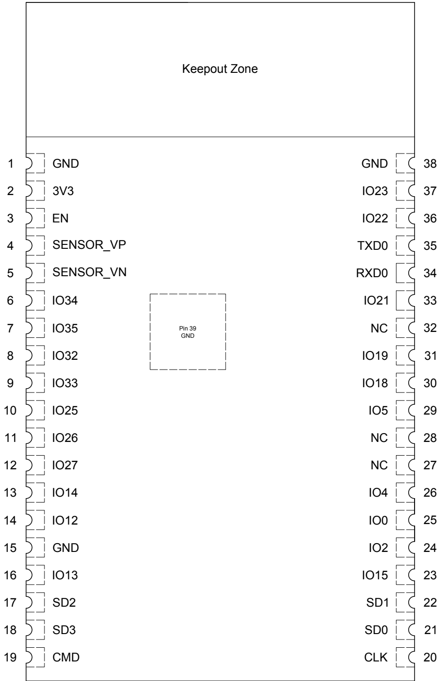
图 1: ESP32-WROVER-B 管脚布局（顶视图）
