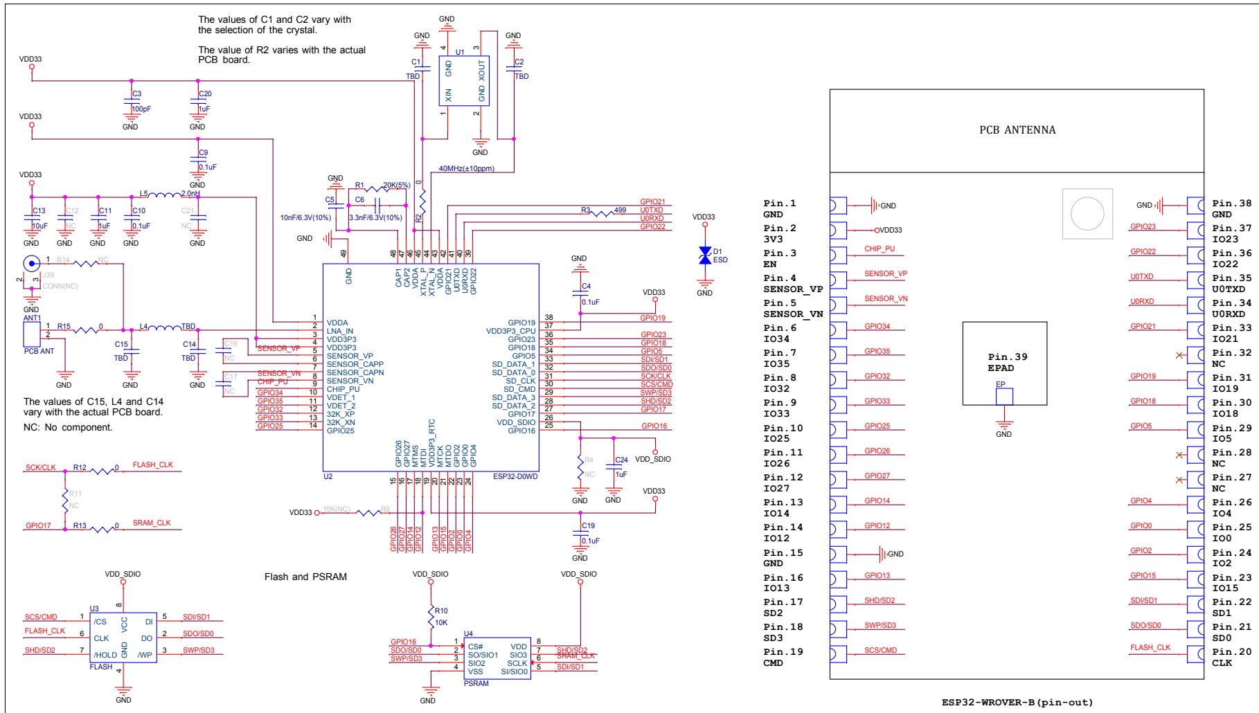
图 5: ESP32-WROVER-B 原理图
