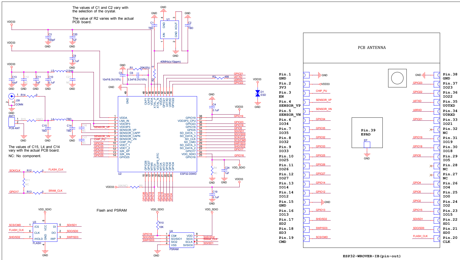
图 6: ESP32-WROVER-IB 原理图
