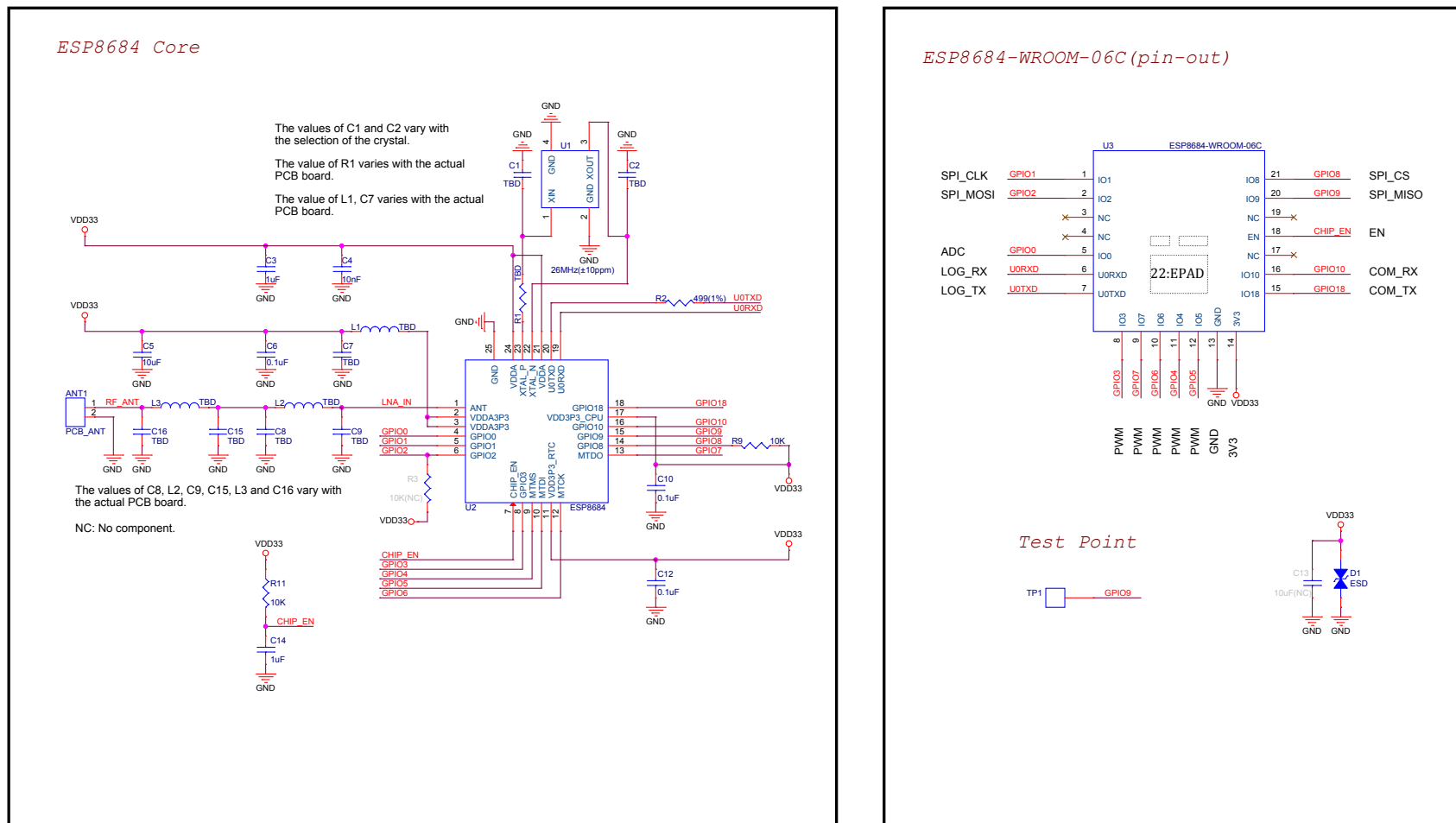
图 4: ESP8684-WROOM-06C 原理图
