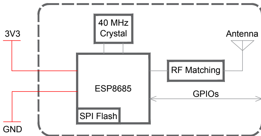
图 2-1. 功能框图
