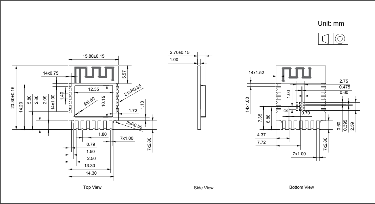
图 10-1. 模组尺寸
