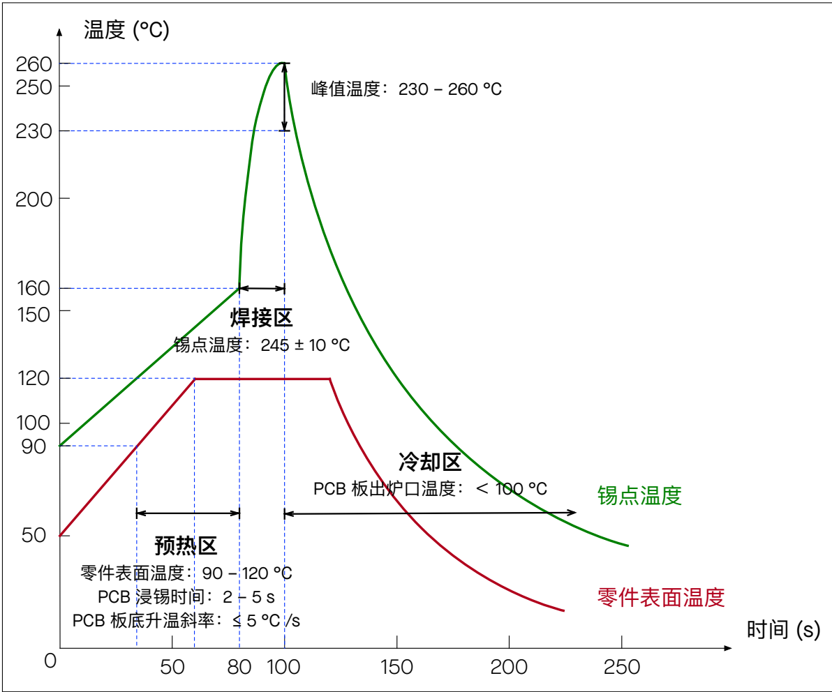
图 12-2. 波峰焊温度曲线
