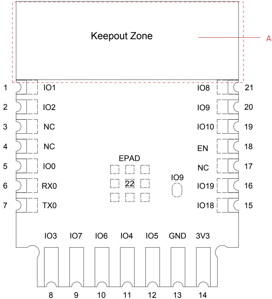
图 3-1. 管脚布局（顶视图）
