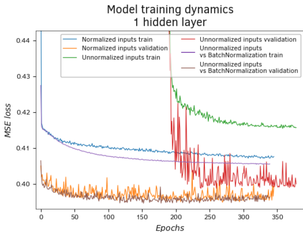
Пакетная нормализация исходных данных (MSE)
