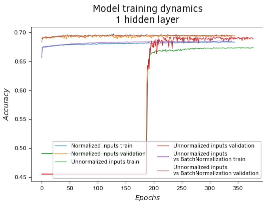
Пакетная нормализация исходных данных (Accuracy)
