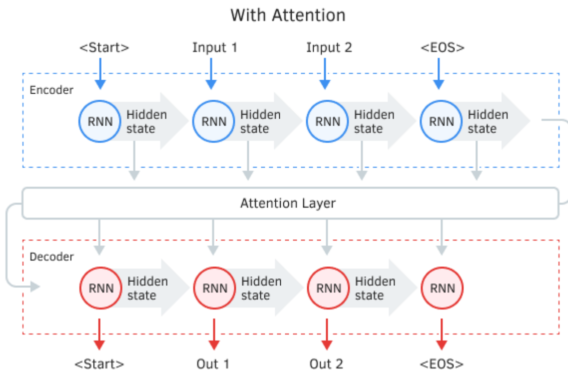
Encoder - Decoder с механизмом внимания
