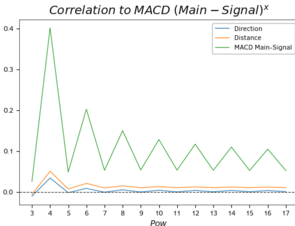
Динамика изменения корреляции значений MACD к ожидаемому движению при возведении показателя в степень
