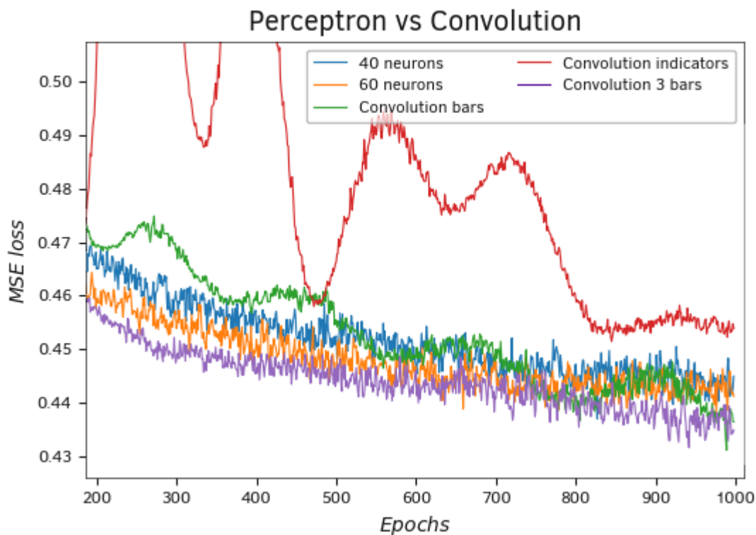
Сравнительный график обучения перцептрона и трех моделей свёрточных нейронных сетей
