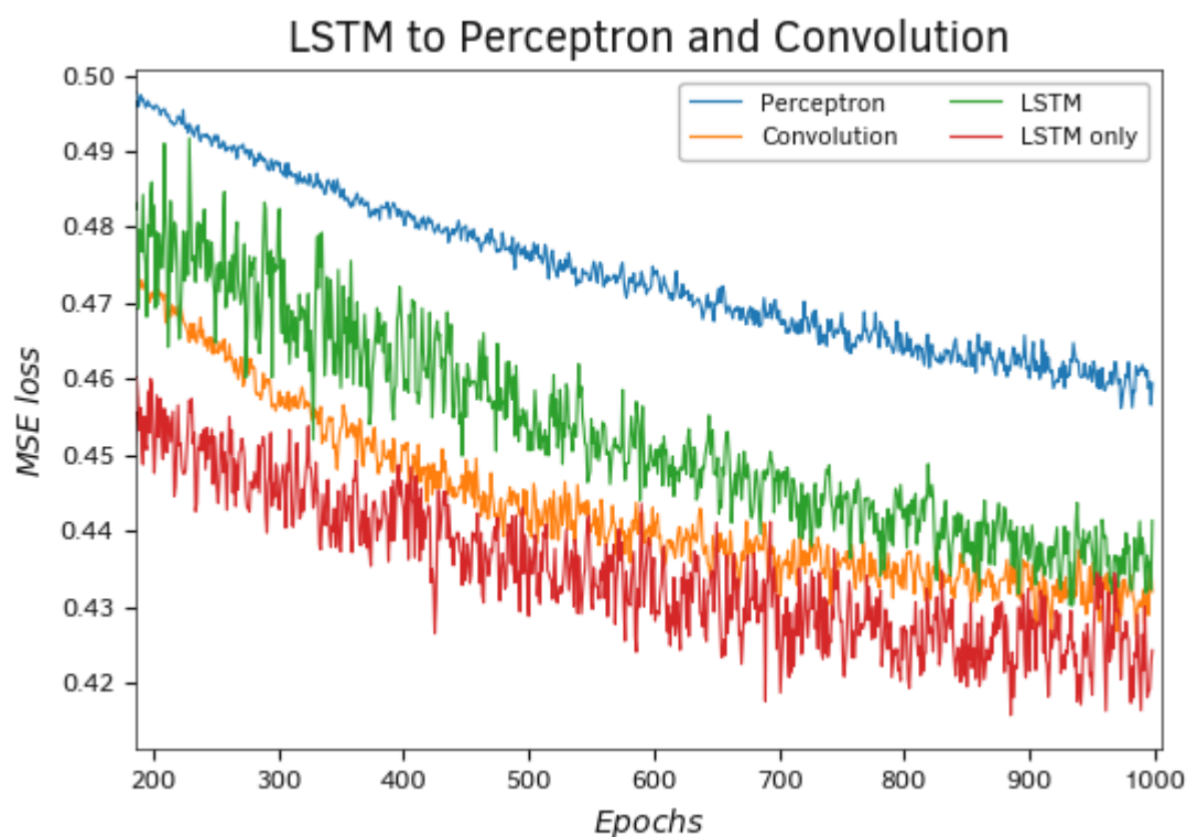
Тестирование модели рекуррентной нейронной сети
