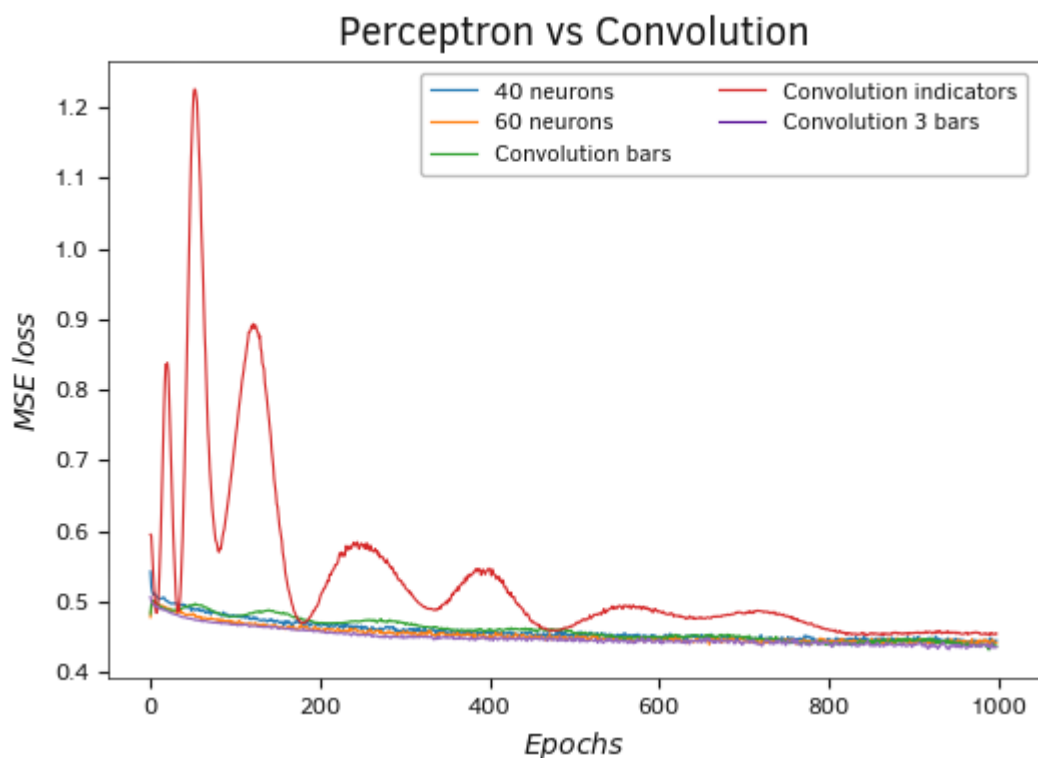
Сравнительный график обучения перцептрона и трех моделей свёрточных нейронных сетей
