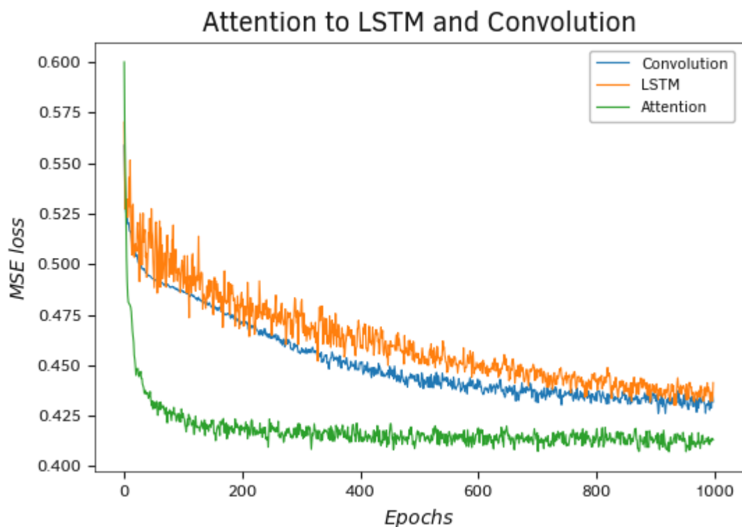
Тестирование модели с использованием блока внимания
