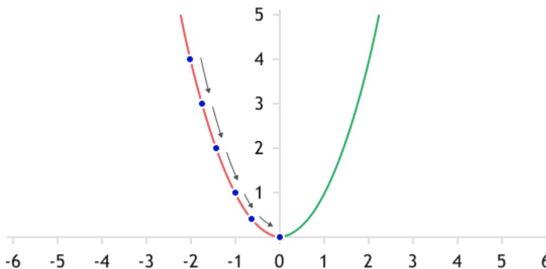
Градиентный спуск
