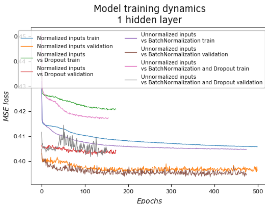
Сравнительное тестирование моделей с Dropout
