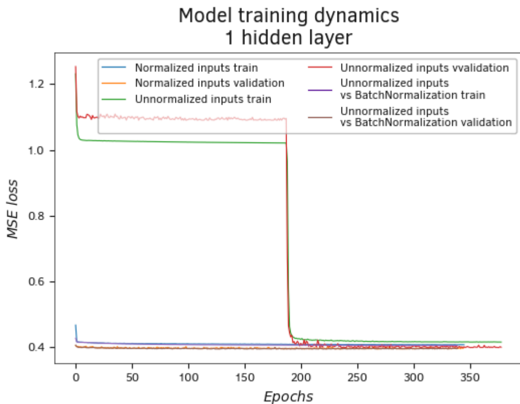
Пакетная нормализация исходных данных (MSE)
