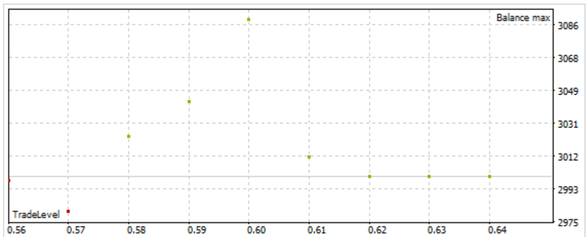
Результаты тонкой настройки параметра принятия решения
