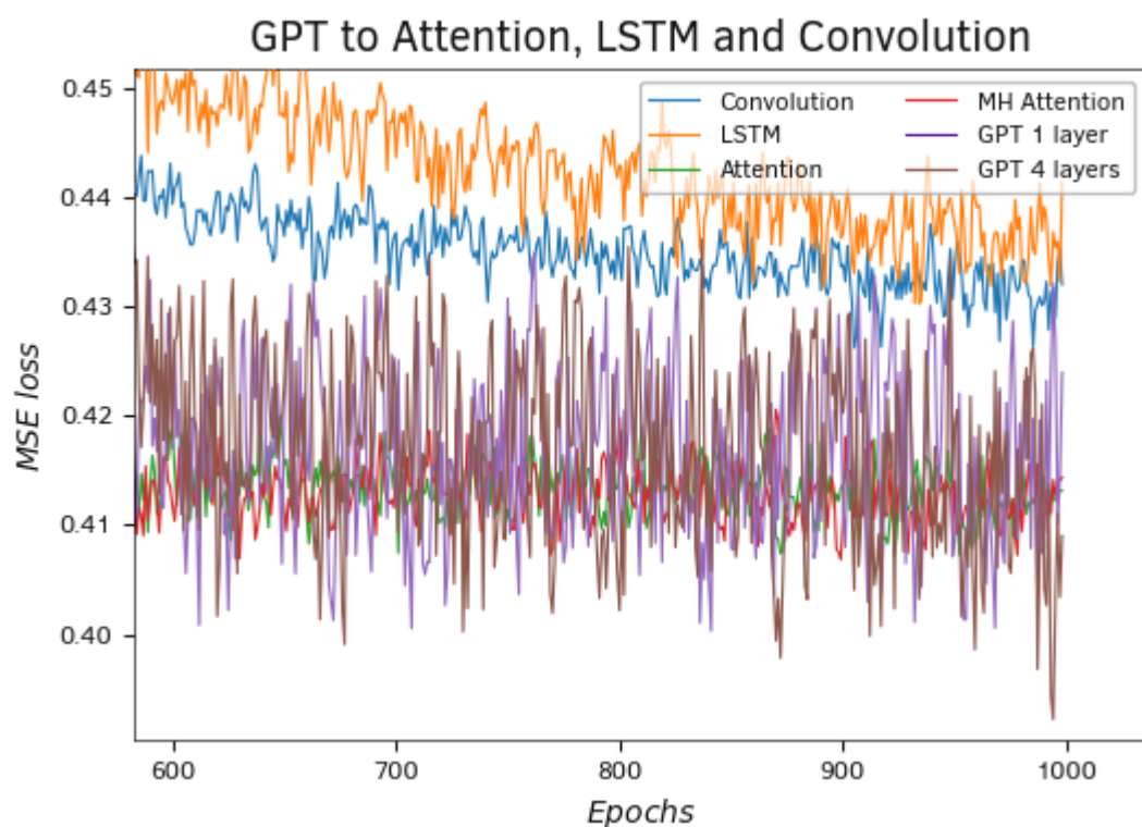
Тестирование модели GPT 4 слоя
