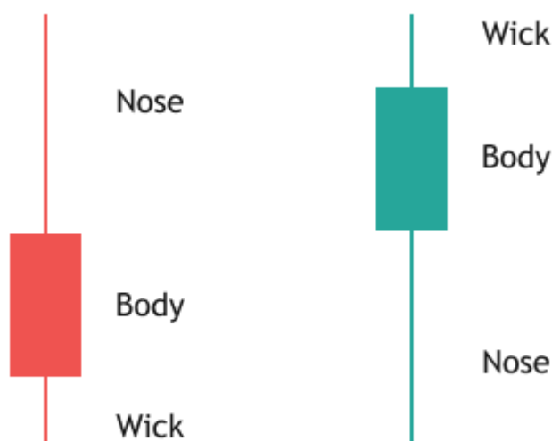
Пин-бар
