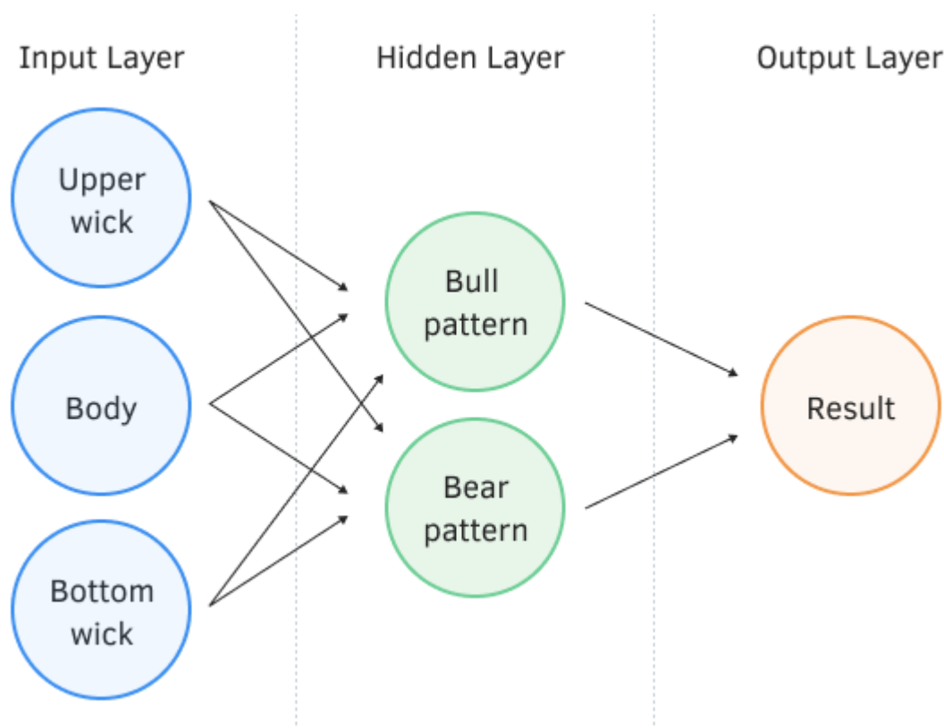
Модель перцептрона
